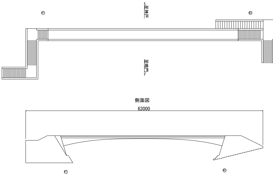
平面図
