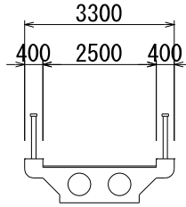
断面図
